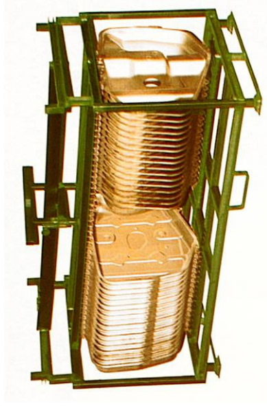
Paleta na lisované plechové diely
